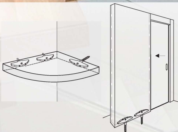
Beschläge für Möbel und Montagen Ferrures pour meubles et montages Fittings for furnitures and mountings
