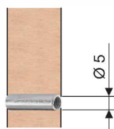
Hülse Stahl verzinkt, M4 Douille acier zingué, M4 Bush galvanized, M4
