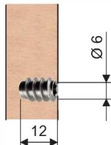
Muffe Stahl M4 Manchon acier M4 Steel socket M4
